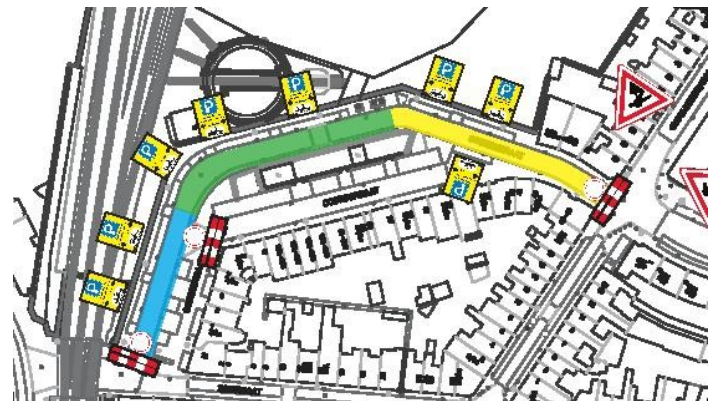
Faseringstekening
