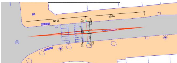
Detailtekening plaatsing paal noordzijde Predikherenstraat
